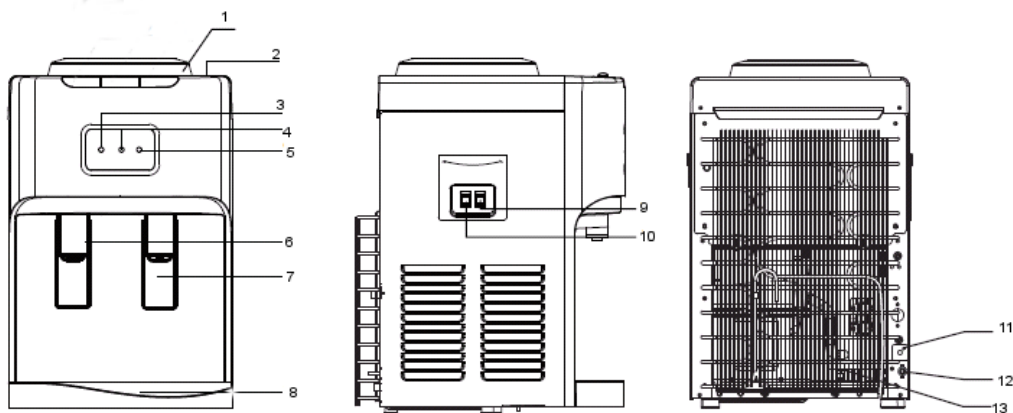
Рисунок 1. Схема аппарата D115
